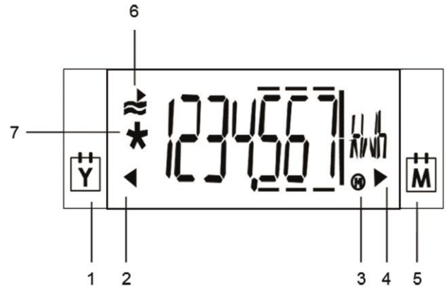
Fig. 6 : Affichage LCD
